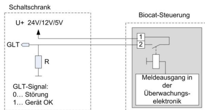
Beispielbeschaltung 2: Einbindung in GLT (Digital-Eingang)
